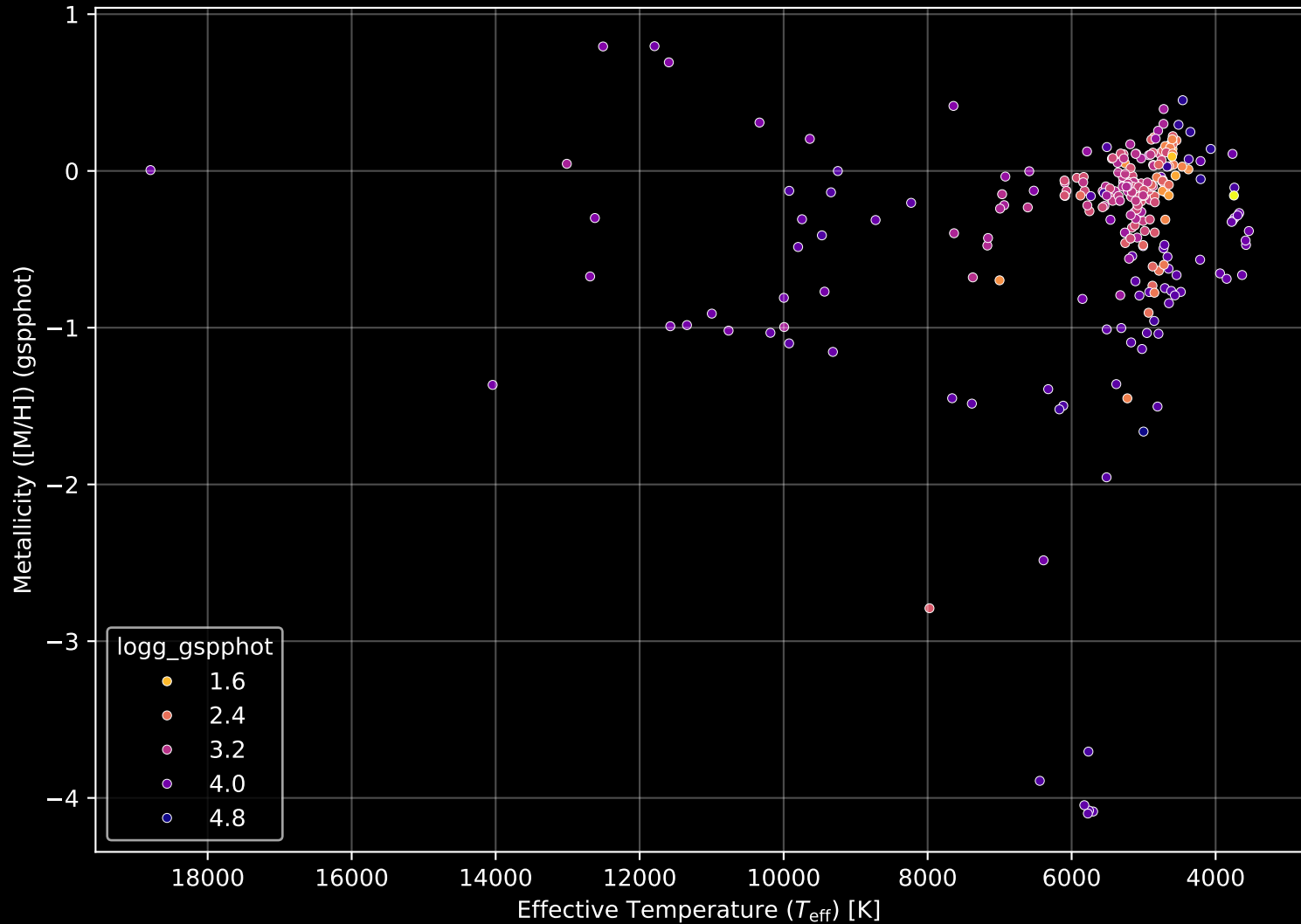
APOGEE DR17 Field: [203+04] Stellar Population Parameters (n= 270)
